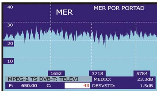
Figura 49.- Función MER por portadora.
