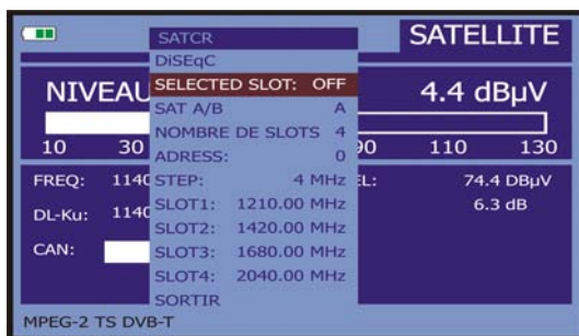
Figure 72.- Écran des commandes SatCR.
